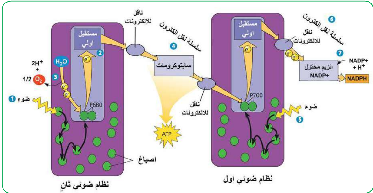
الشكل (6) تفاعلات المسار الإلكتروني اللاحلقي
